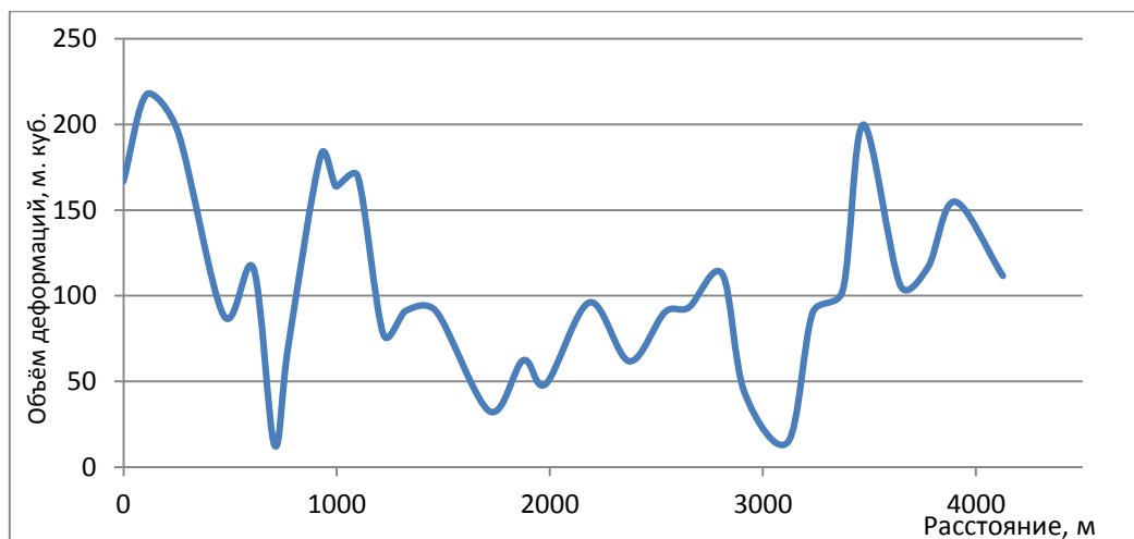
Рисунок 1 – Деформации русла реки Томи от стадиона ТГУ до гидрологического поста Томск-пристань за 2014–2017 гг.
