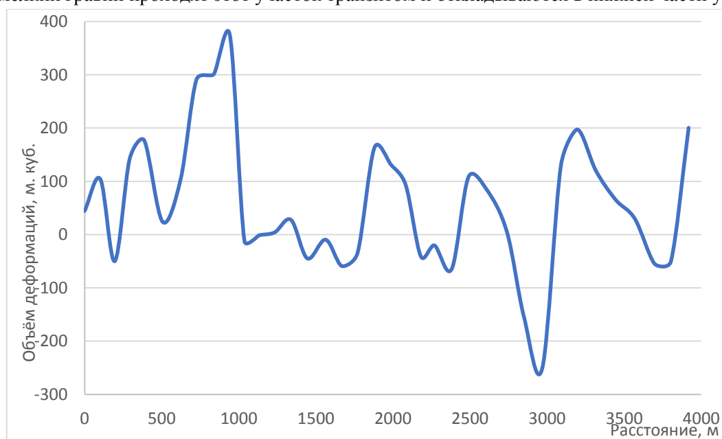
Рисунок 2 – Деформации русла реки Томи от стадиона ТГУ до гидрологического поста Томск-пристань за 2018 г.
