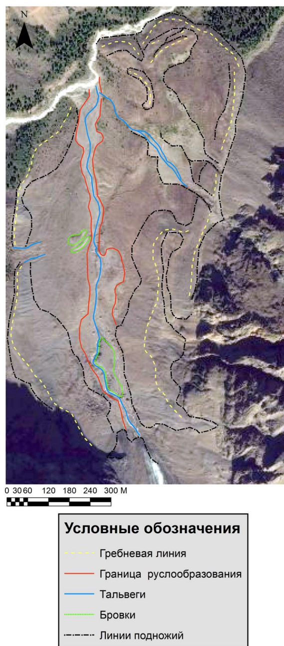
Рисунок 1 – Структурные линии перигляциального рельефа ледника Малый Актру
