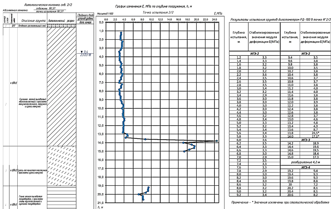
Рисунок 2 – Результаты обработки данных дилатометра рядом со скважиной 2
