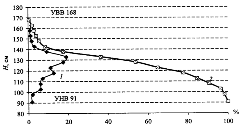
Рисунок 2 – Кривые повторяемости (частоты) (1) и продолжительности (обеспеченности) (2) уровня воды в л. Курчанского – г. Темрюк за 1966-2018 гг. [8]
