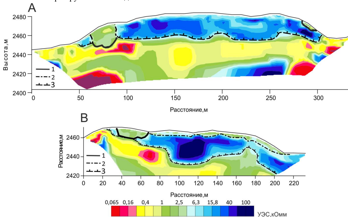
Рисунок 2 – Геоэлектрические разрезы ГМКО в долине р. Джело:
