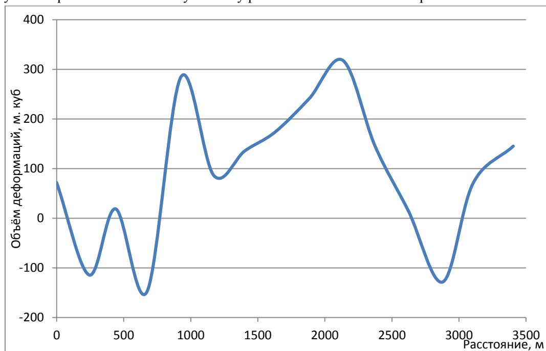
Рисунок 3 – Деформации русла реки Томи от гидрологического поста Томск-пристань до истока Татарской протоки за 2014–2018 гг.
