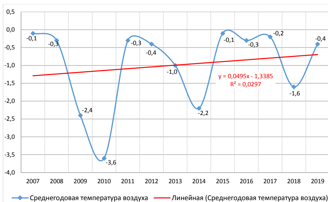
Рисунок 1 – График среднегодовой температуры воздуха (°C) по данным метеостанции города Нижневартовска за 2007-2019 гг.
