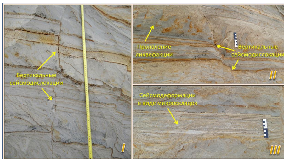
Рисунок 2 – Различные сейсмодетформации в позднеплейстоценовых аллювиальных осадках 20-м Надымской террасы; окрестности г. Надым. Фото из архива В.С. Шейнкмана и Г.В. Матышака. Пояснения в тексте
