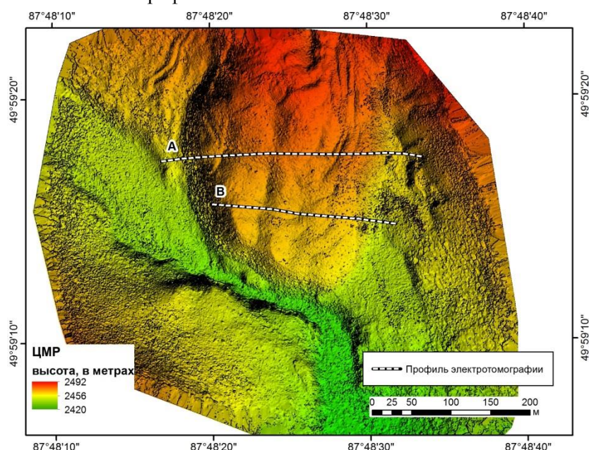
Рисунок 1 – Цифровая модель рельефа ГМКО и прилегающей территории и линии профилей электротомографии
